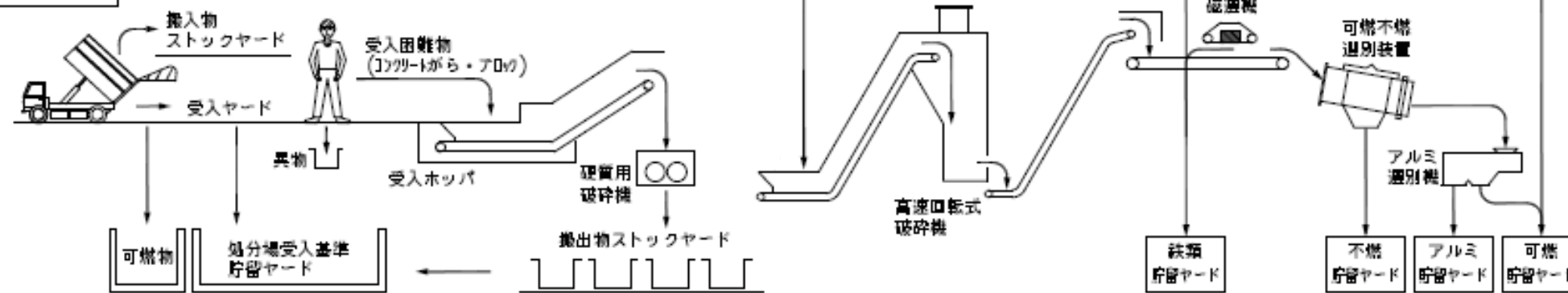
リサイクルセンター 処理フロー (一例)
