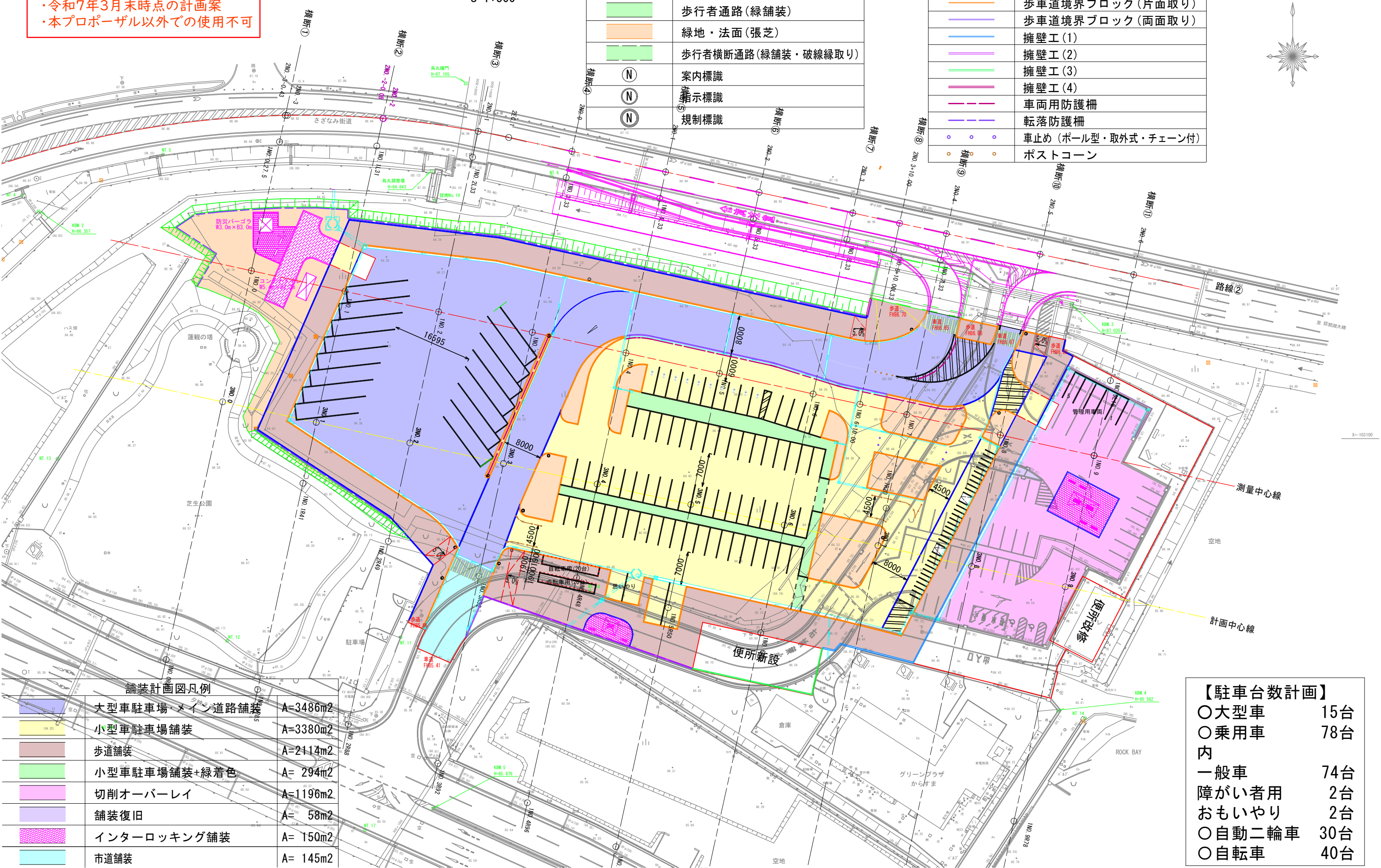
計画平面図 S=1:500
