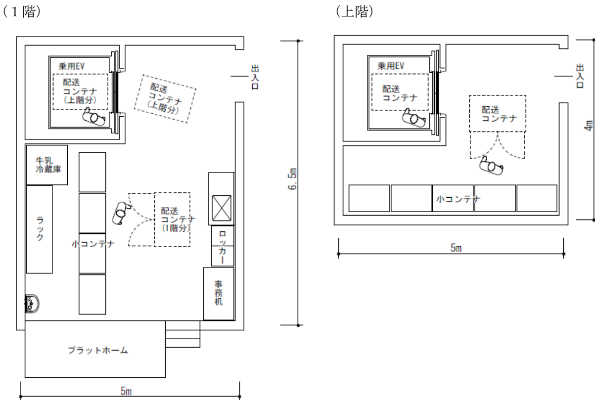
図表30 配膳室配置例(参考図)
