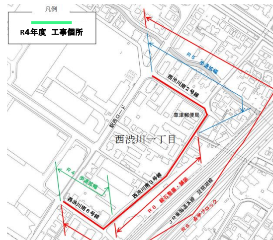
▲西渋川南3号線歩道改良工事施工 位置図
