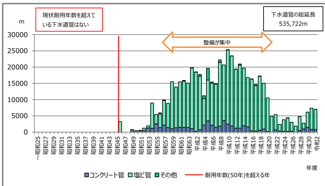
図 17 下水道施設の年度別整備状況
