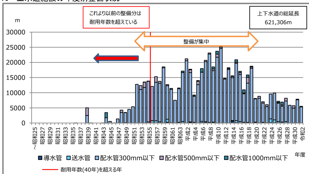
図 16 上水道施設の年度別整備状況
