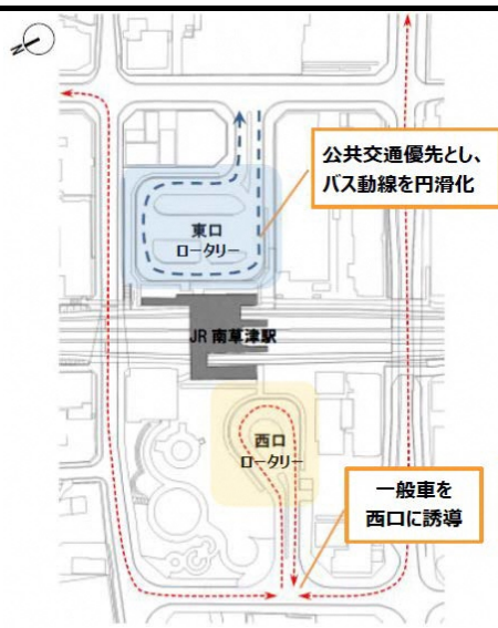
図 南草津駅前広場の交通誘導（案）
