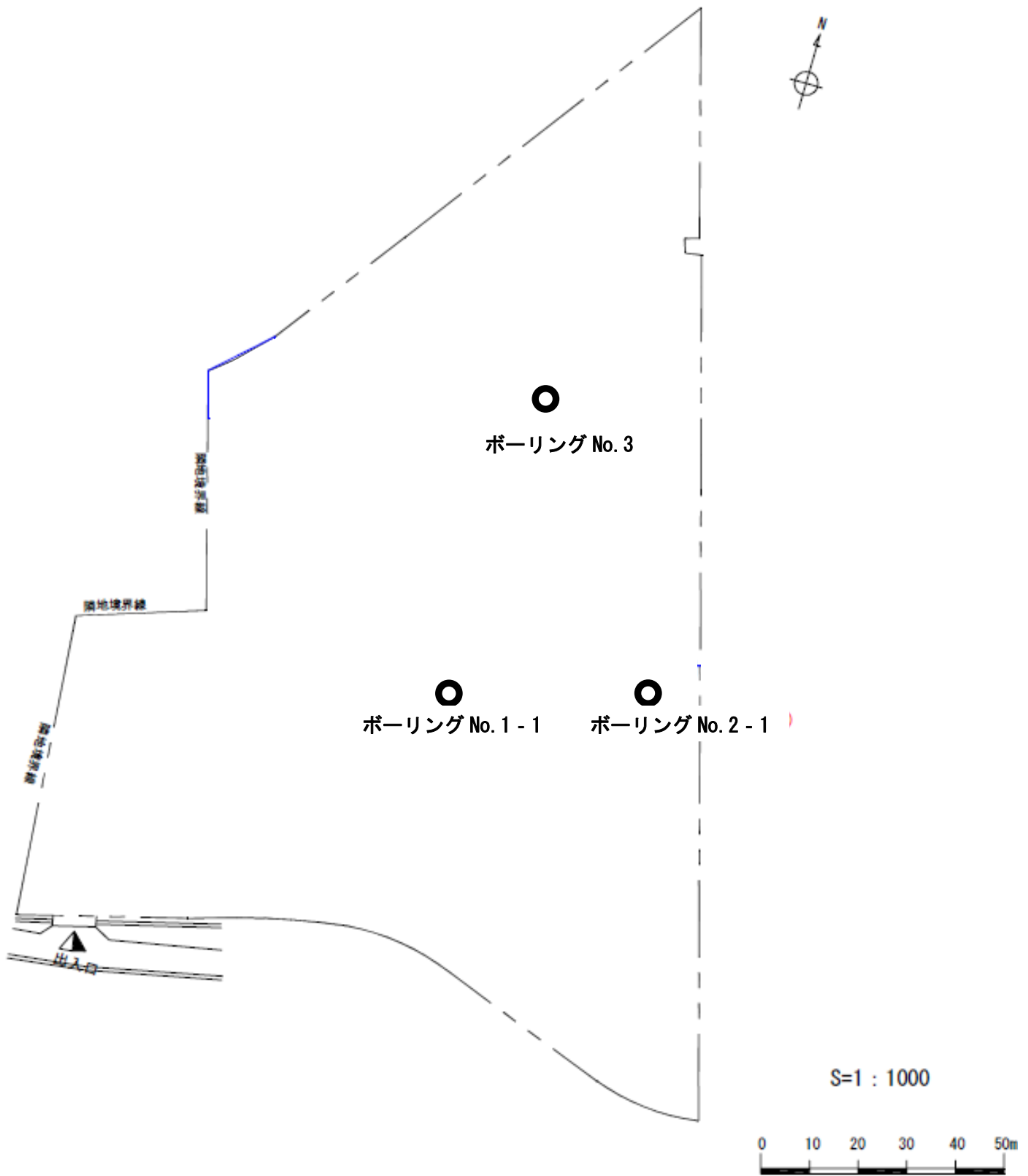
ボーリング調査地点位置図
