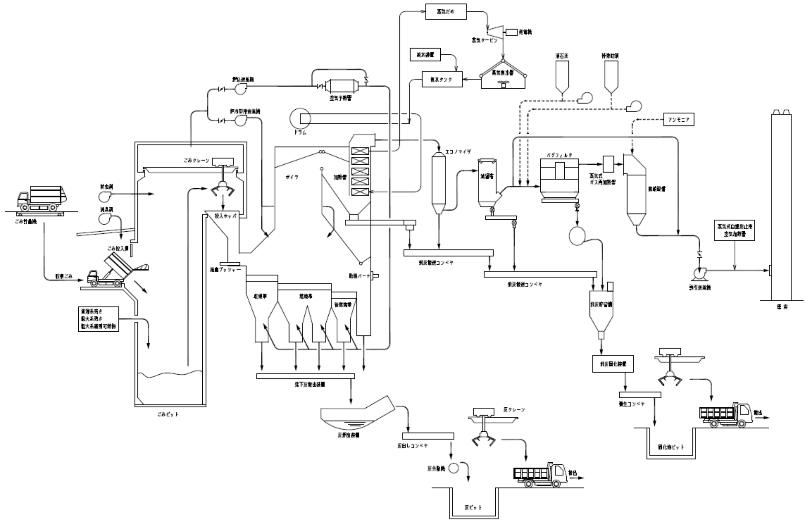
熱回収施設 処理フロー（一例）
