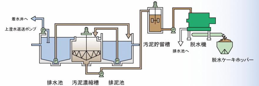
排水排泥処理設備
