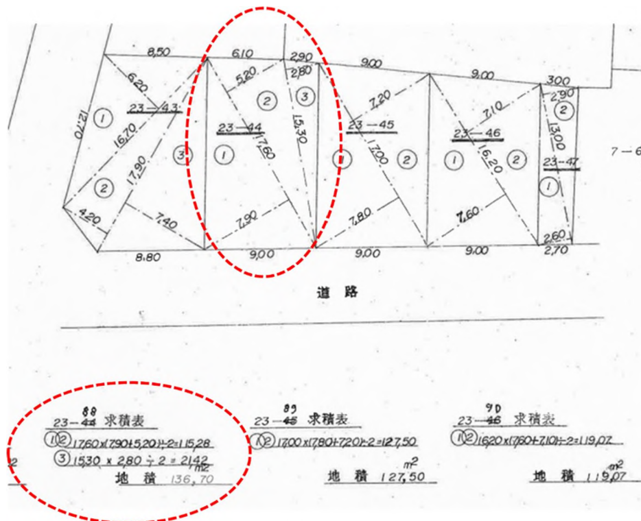
地積測量図
