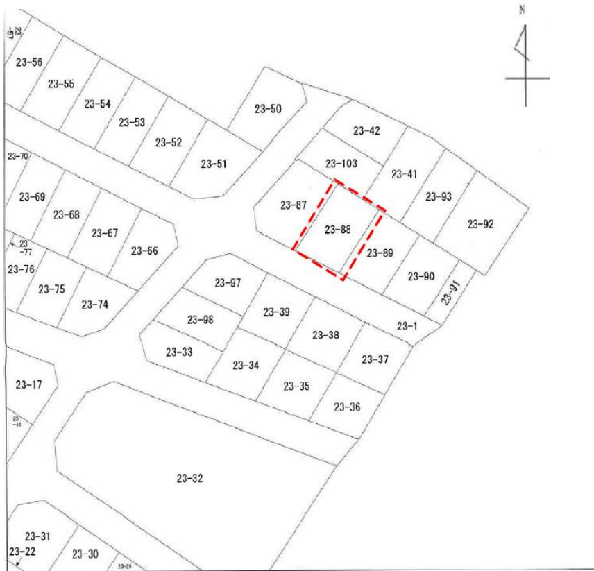
地積測量図
