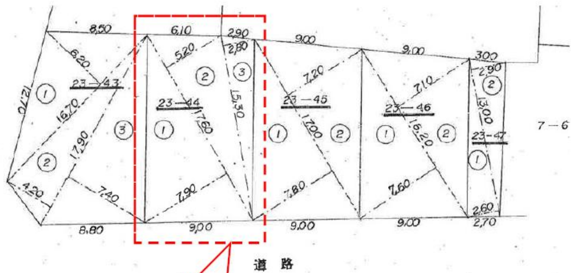
地積測量図
