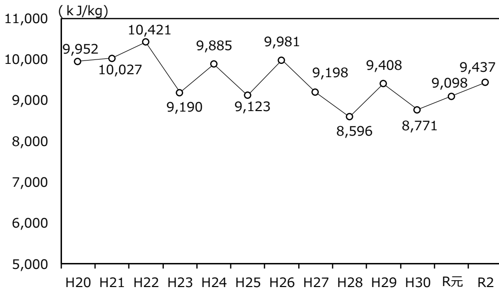
図 2-6 低位発熱量の推移
