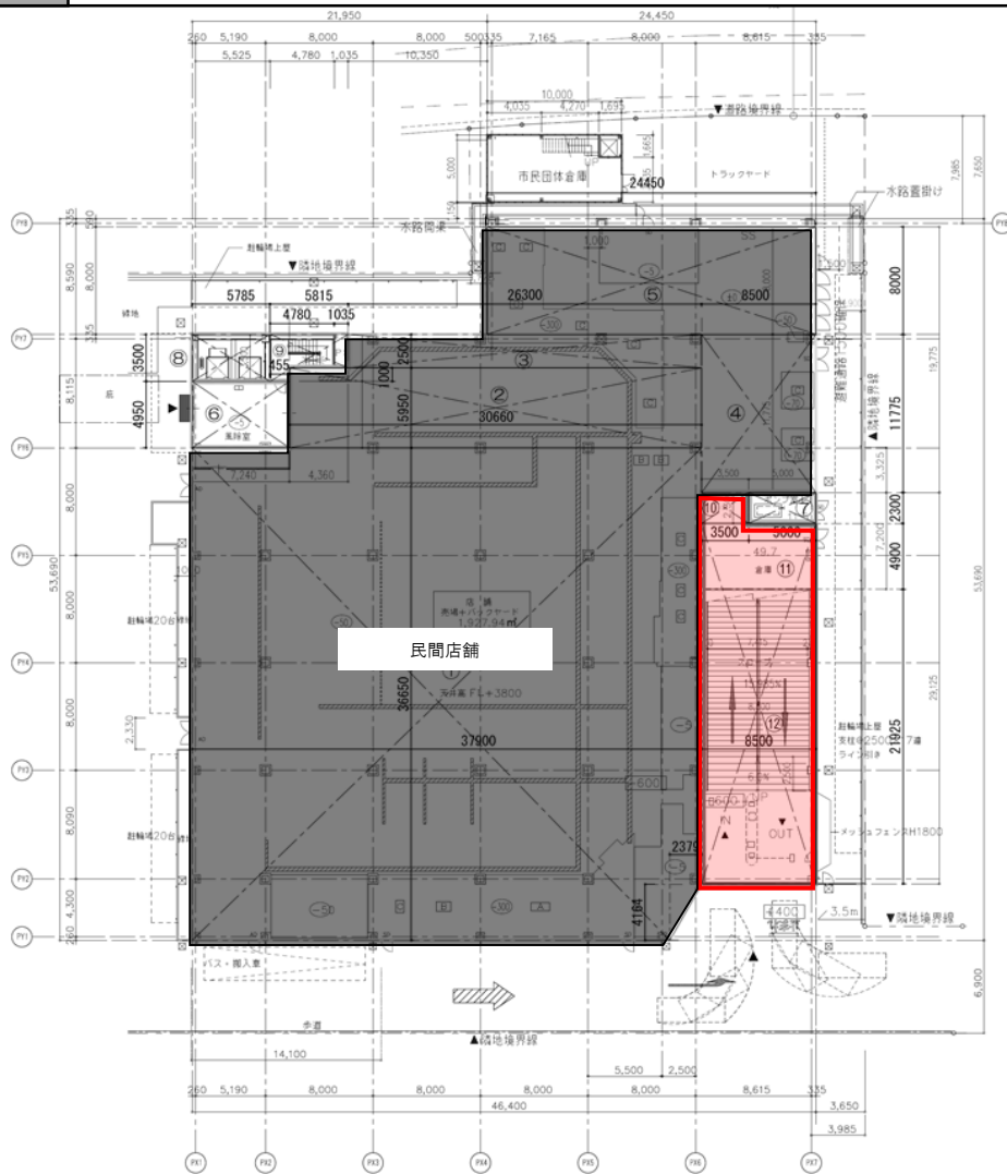
1階平面図
