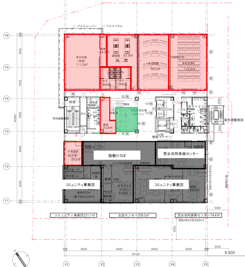
5階平面図
