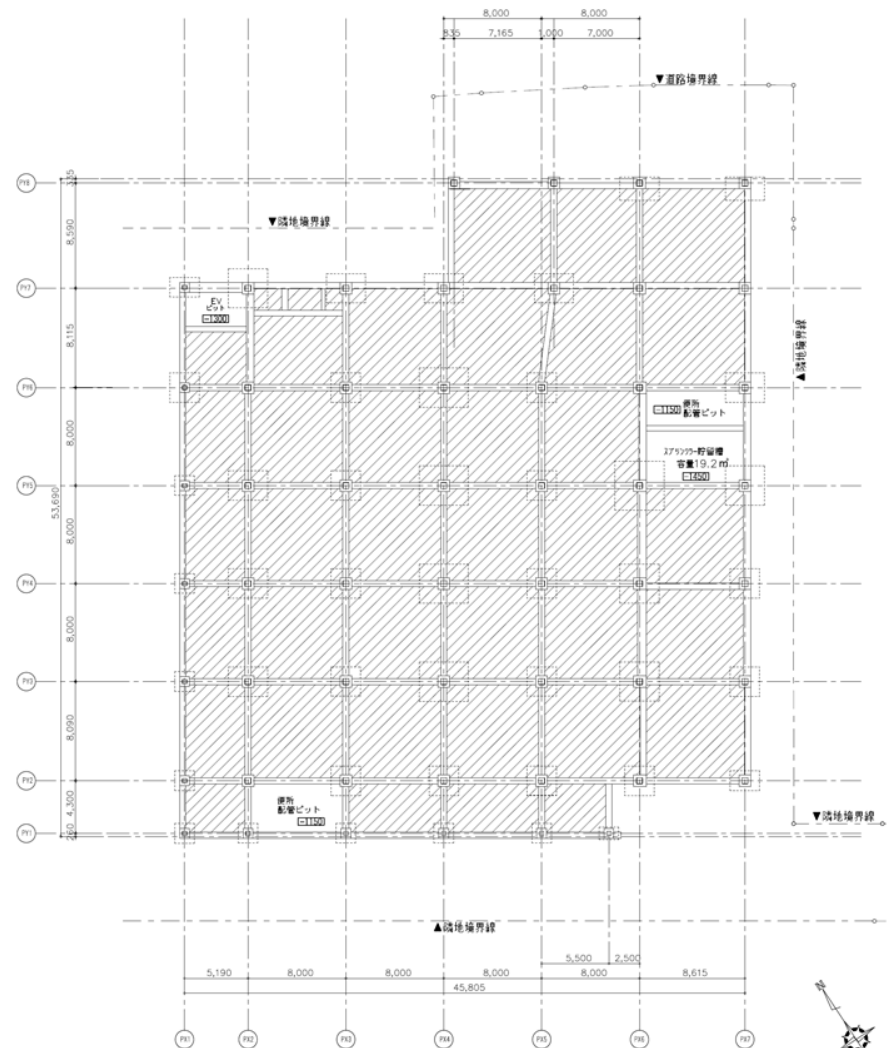
ビット平面図
