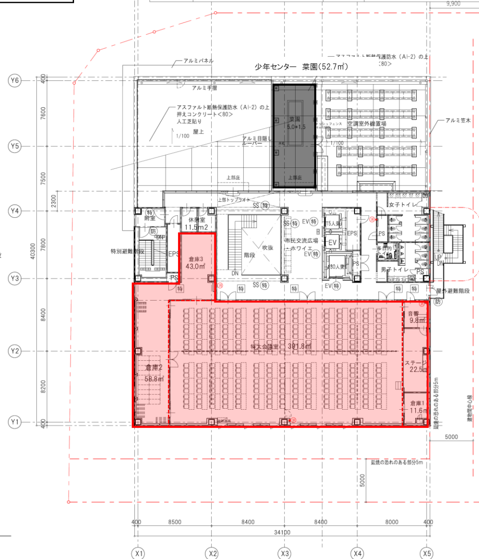
6階平面図
