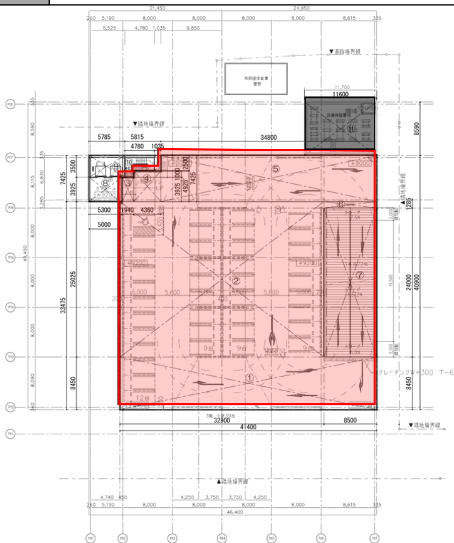
3階平面図
