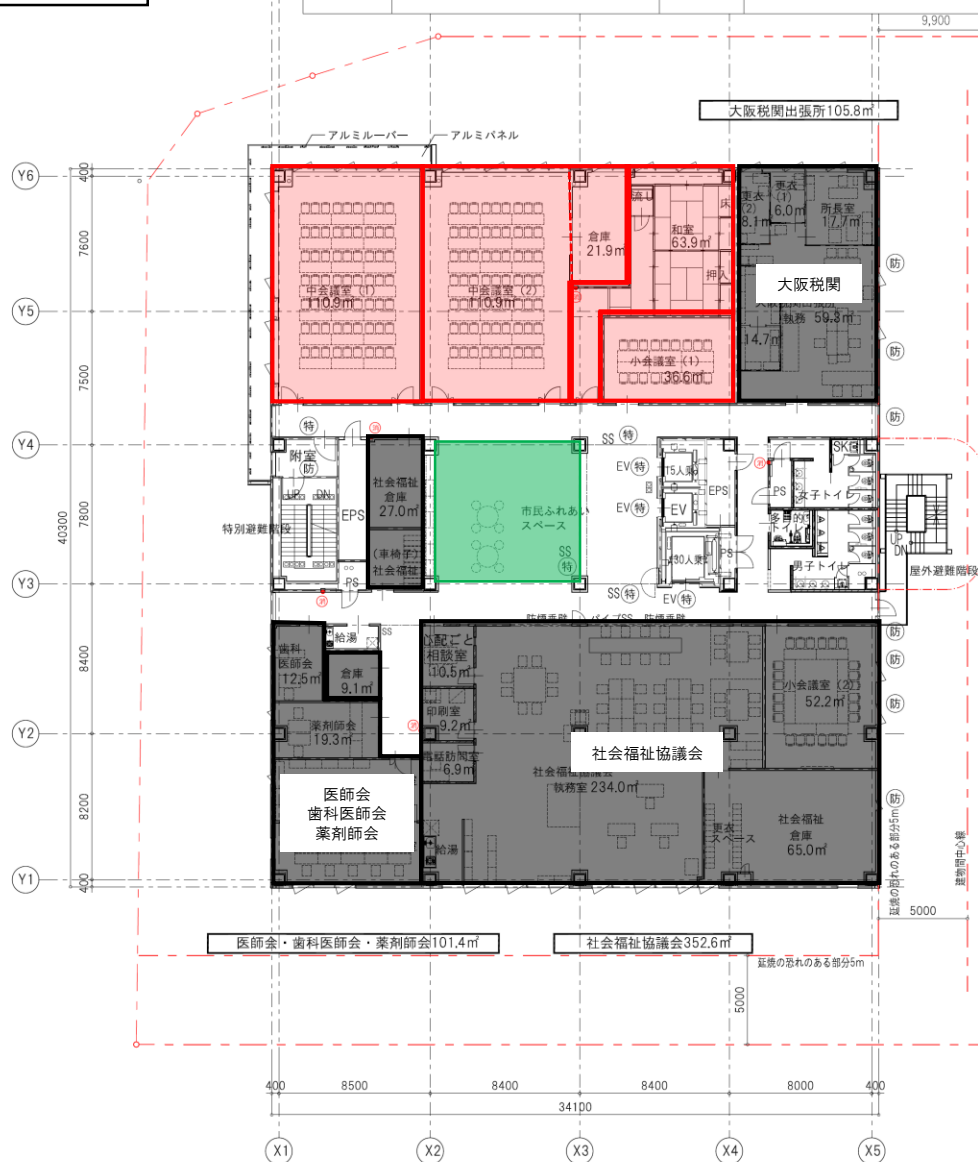
4階平面図
