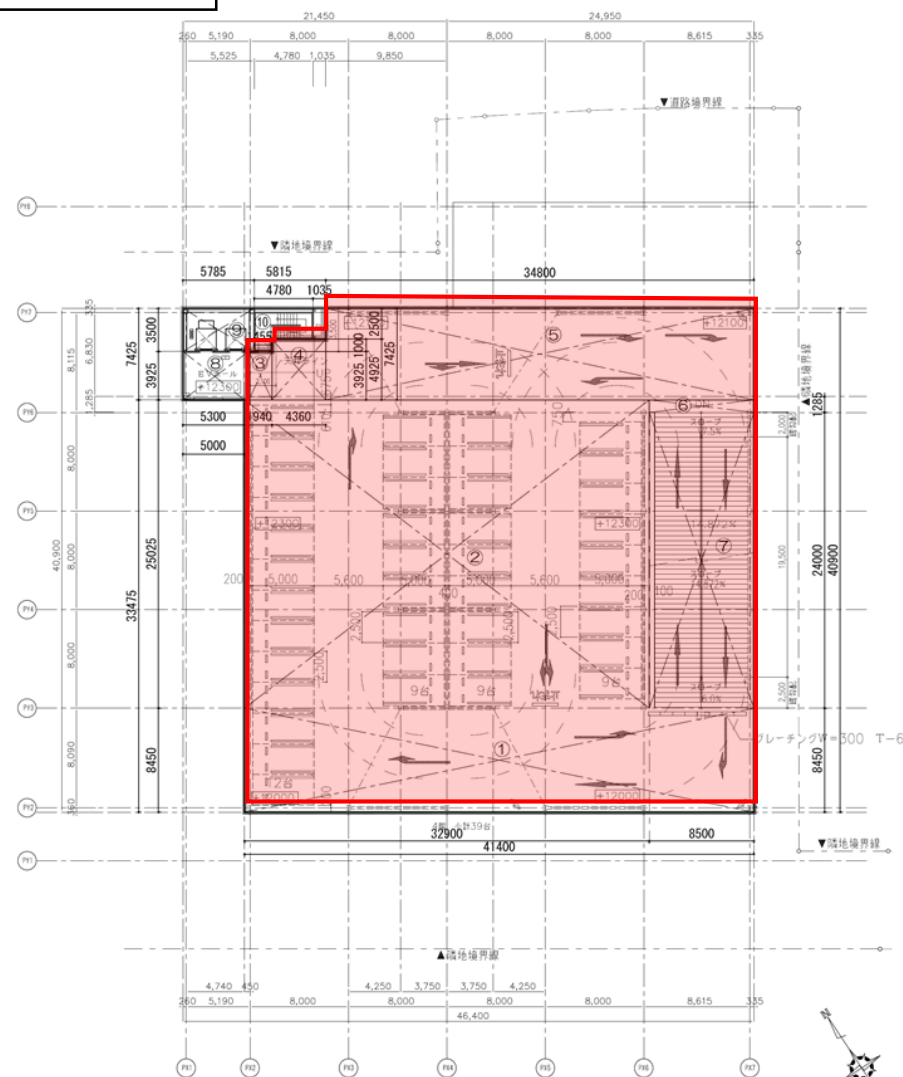
4階平面図
