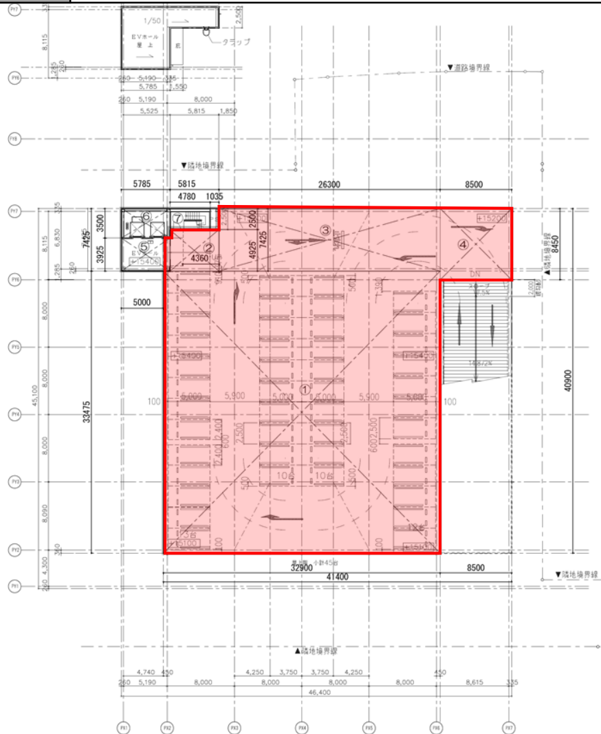
R階平面図
