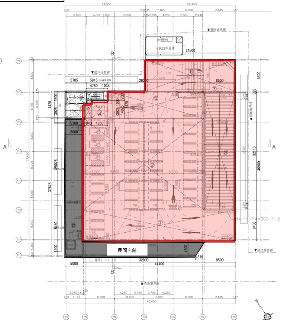
2階平面図
